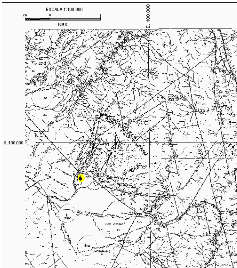
Tomado de: Geología de Superficie de la Creole Petroleum Corporation, Hoja E-4, 1963.
